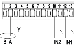
Сх. 7: Съемная клеммная колодка 13 полюсов: цифровые входы и MODBUS
